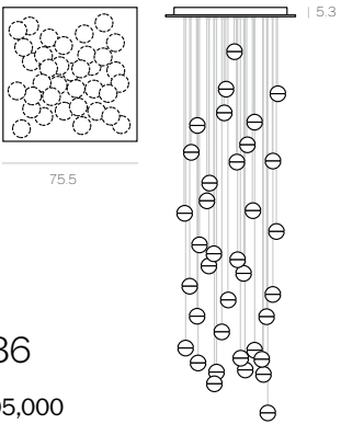
14.36 Round ¥4,305,000 全長 max.300cm(現場調整不可) シェード Ø:10.2cm ×36 フランジ Ø:75.5 H:5.3cm ホワイト色塗装 重量 約 83.5kg
