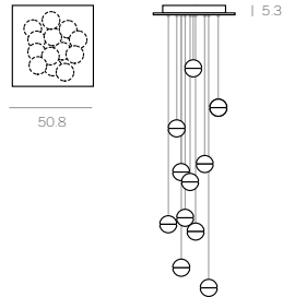
14.11 Square ¥1,316,000 全長 max.300cm(現場調整不可) シェード Ø:10.2cm ×11 フランジ W:50.8 D:50.8 H:5.3cm ホワイト色塗装 重量 約 29.5kg
