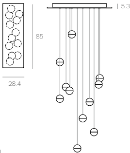
14.11 Rectangle ¥1,316,000 全長 max.300cm(現場調整不可) シェード Ø:10.2cm ×11 フランジ W:85 D:28.4 H:5.3cm ホワイト色塗装 重量 約 29.5kg
