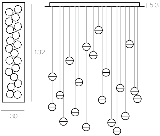
14.20 Rectangle ¥2,392,000 全長 max.300cm(現場調整不可) シェード Ø:10.2cm ×20 フランジ W:132 D:30 H:5.3cm ホワイト色塗装 重量 約 63kg
