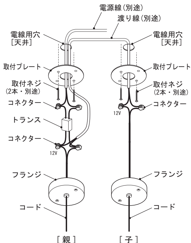
図6 ※1台のトランスに器具2台を接続する場合
