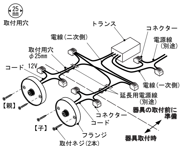
図4 ※1台のトランスに器具2台を接続する方法
