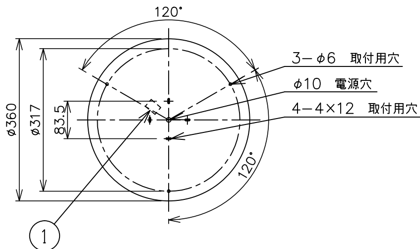
取付面図
