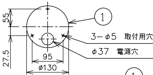
取付面図
