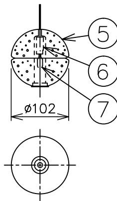
灯具部分の詳細図
