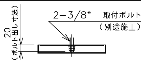
取付部詳細
