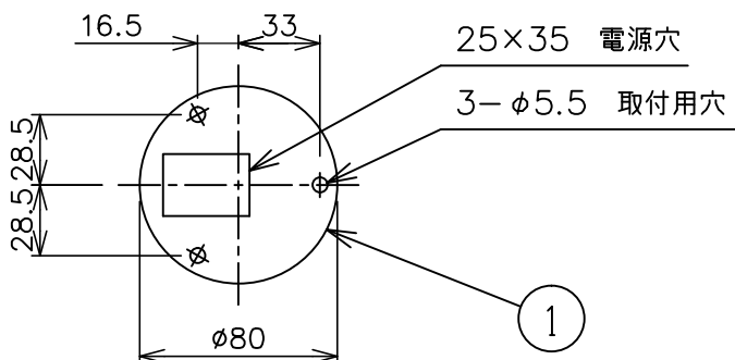
取付面図
