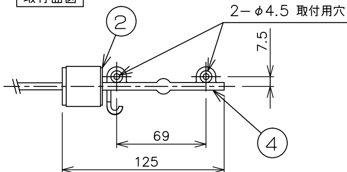
取付面図
