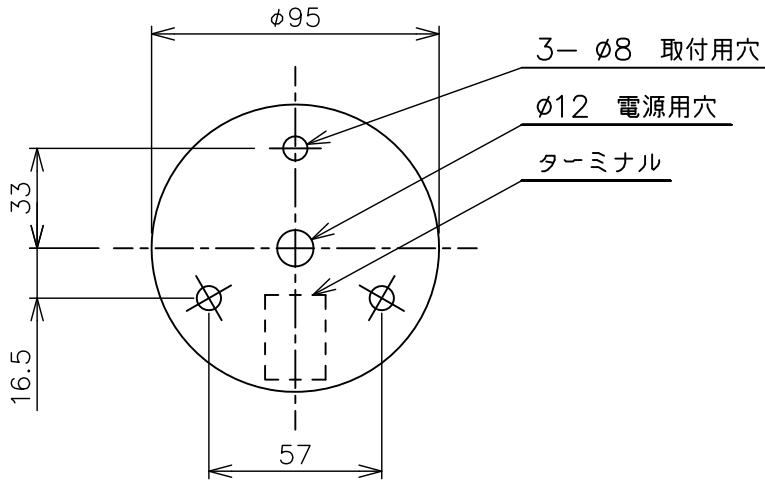
取付面図
