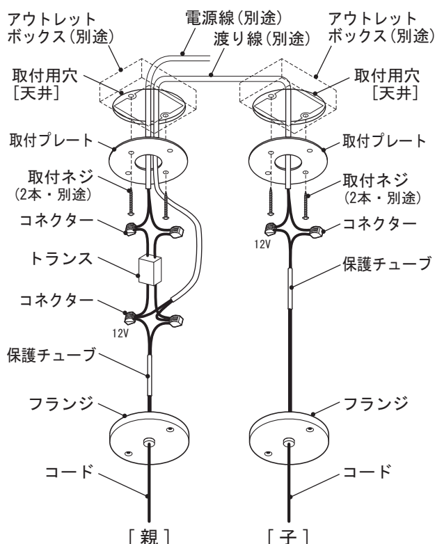
図 5 ※1 台のトランスに器具 2 台を接続する場合 [既設の引掛ローゼットの取付用穴を利用した取付方法]
