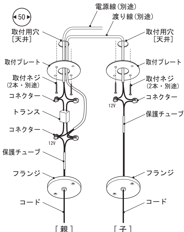
図 4 ※1 台のトランスに器具 2 台を接続する場合 [一般的な取付方法]
