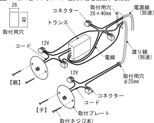
図1 ※1台のトランスに器具2台を接続する方法
