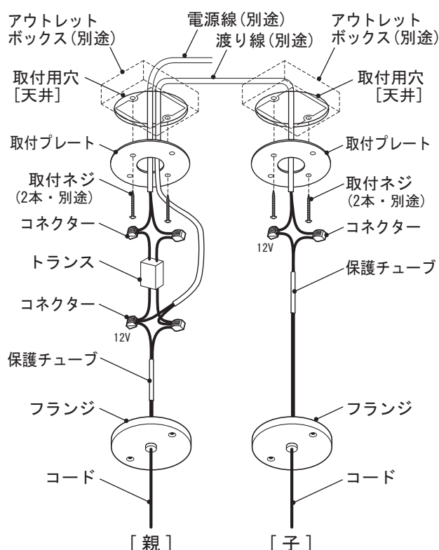
図 5 ※1台のトランスに器具2台を接続する場合 [既設の引掛ローゼットの取付用穴を利用した取付方法]
