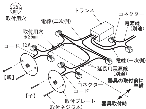
図7 ※1台のトランスに器具2台を接続する方法
