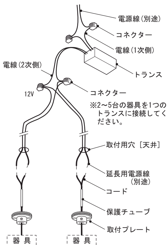
図 9 ※ 1 台のトランスに器具 2 台を接続する場合
